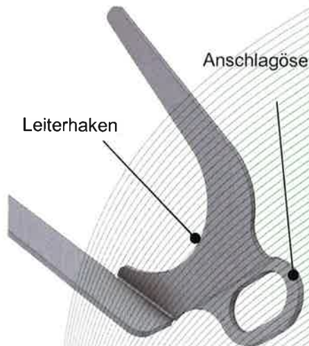
Bild 1: Aufbau Sicherheitsdachhaken
